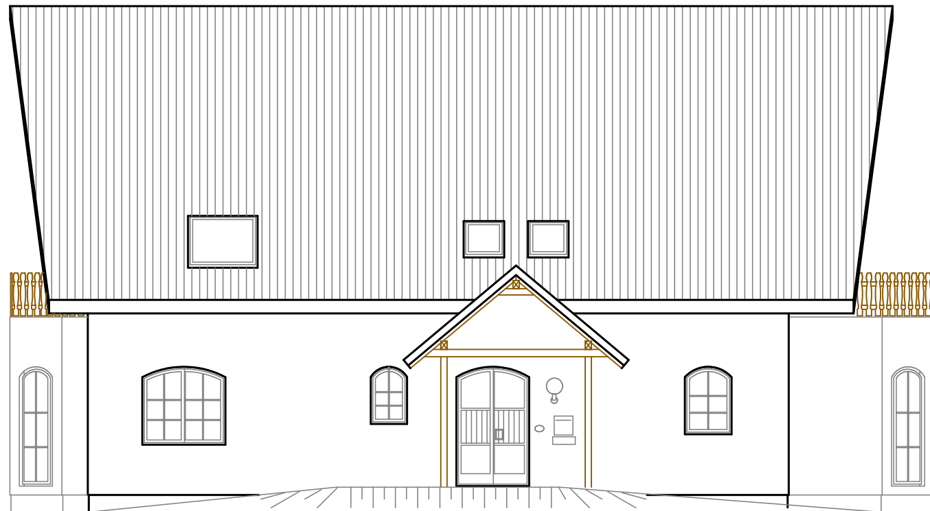
FRONTANSICHT
